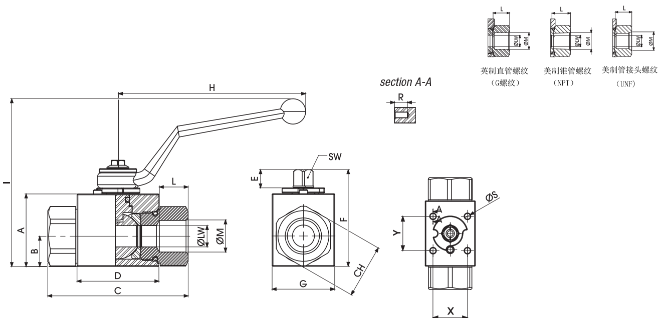
英制直管螺纹（G螺纹）球体尺寸及工作压力 带固定安装孔 DIN/ISO5211
