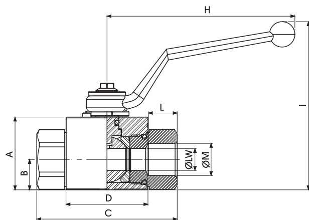
英制直管螺纹（G螺纹）球体尺寸及工作压力
